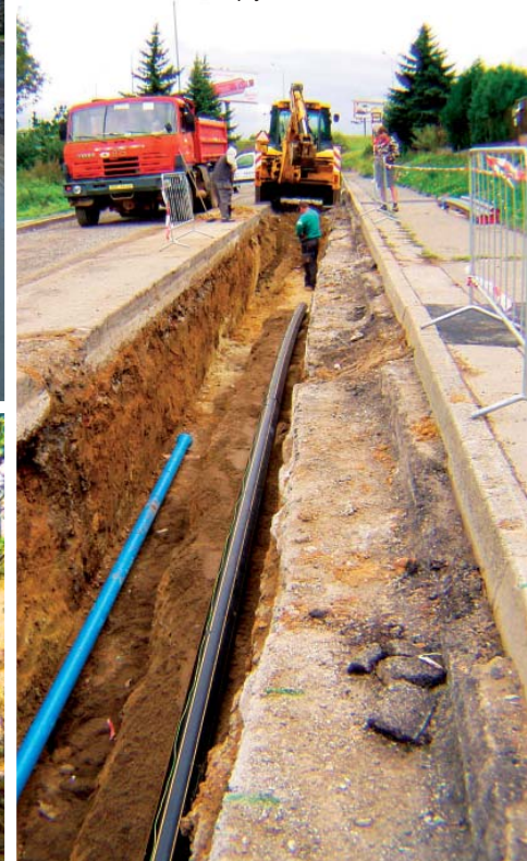
Pokládka vodovodu a plynovodu v ulici Ke Smíchovu
